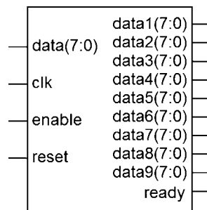
Figure 8 Module SIPO.
