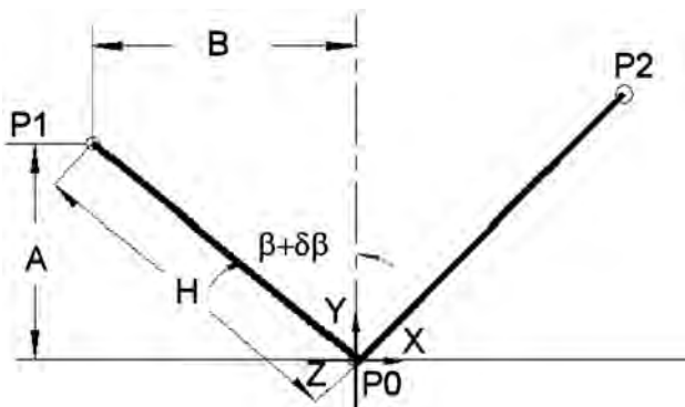
FIGURA 3. Posiciones de la fuente y el punto donde el haz incide sobre el DC, para el caso en que el instrumento se ha girado un ángulo \delta\beta (nuevamente el giro se ha exagerado). El eje Z del sistema coordenado apunta hacia fuera del dibujo y además el punto P_0 coincide con el origen del sistema de referencia.
