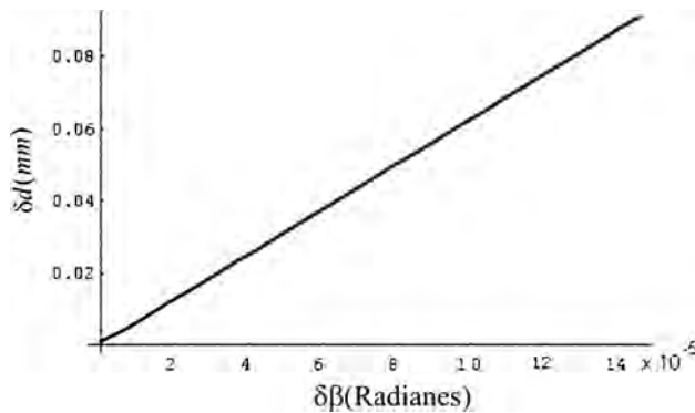
FIGURA 5. Desplazamiento del haz en función de la inclinación del instrumento, para un ángulo \beta=75^\circ .
